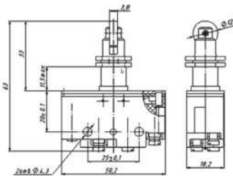
МП45-21-20711-00УХЛ3
