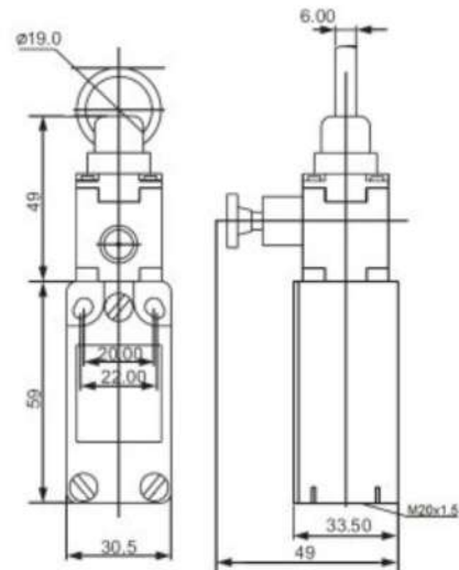
ВП19М21ВХТ1-65У2.1Х тросовый
