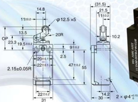
ВП31М21Б251-66У2.11(12,21,22) поворотный рычаг с роликом
