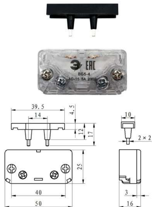
ВБ5-4-00УХЛ3
