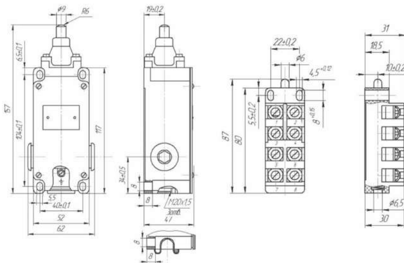
ВП19М21Б4Х1-67У2.1Х, толкатель
