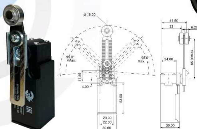
П19М21Б292-65У2.18(10,19,28) поворотный регулируемый рычаг с роликом
