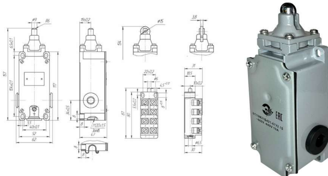
ВП19М21Б421-67У2.1Х, толкатель с роликом
