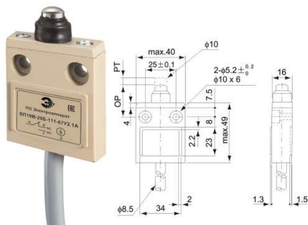
ВП19М20Б111-67У2.1А, толкатель
