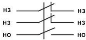
1НО+2НЗ (11)
