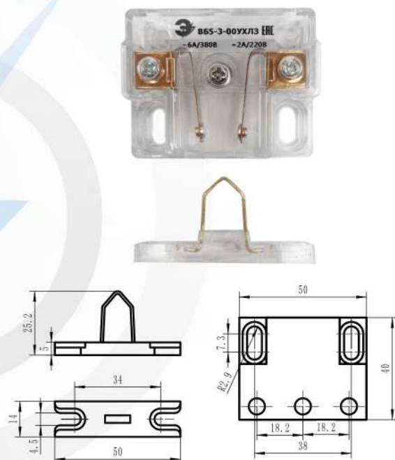
ВБ5-3-00УХЛ3
