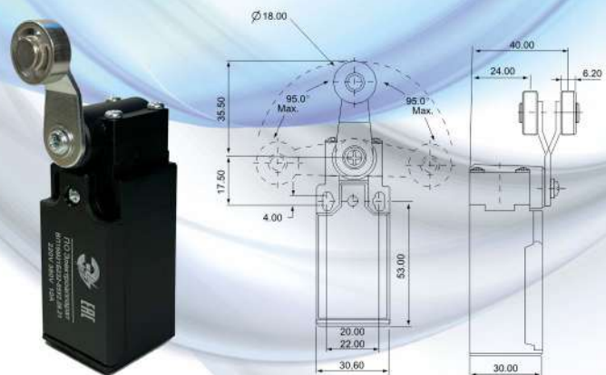
ВП19М21Б292-65У2.18(10,19,28).33А поворотный регулируемый рычаг с регулируемым по выносу резиновым колесом
