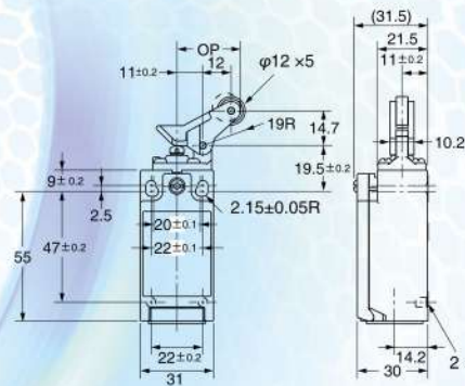
ВП31М21Б241-66У2.11(12,21,22) обратный рычаг с роликом
