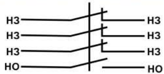
ВП19М21А410-20УЗ.1Б
