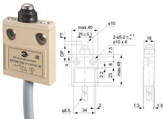
ВП19М20Б111-67У2.1А, толкатель
