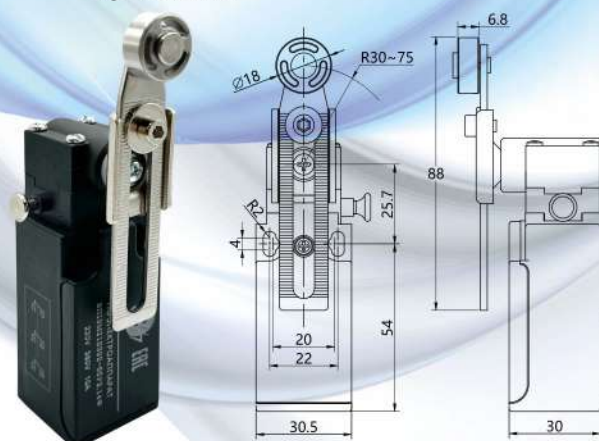
ВП19М21Б392-65У2.11(12,14) Ф поворотный регулируемый рычаг с роликом
