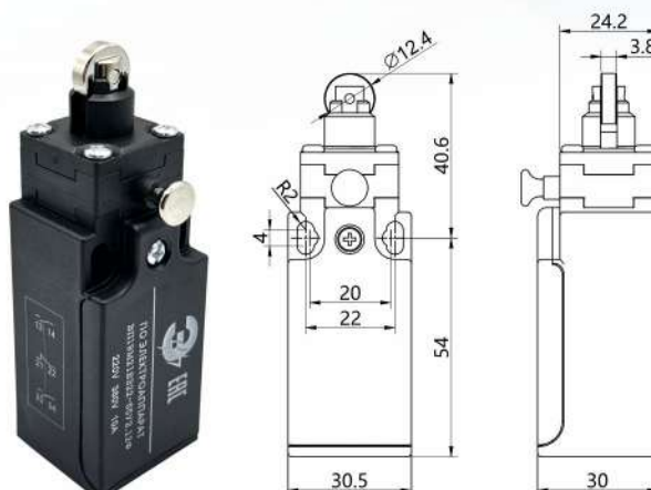
ВП19М21Б322-65У2.11(12,14)Ф толкатель с роликом
