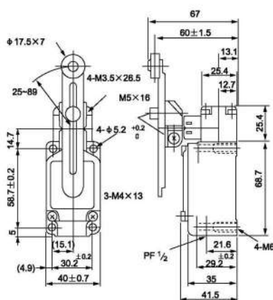
ВП15К21А291-66У2.3 поворотный регулируемый рычаг с роликом
