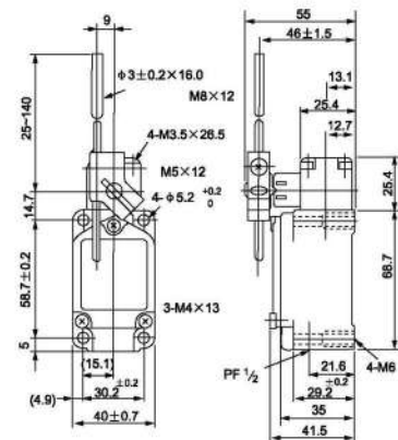
ВП15К21А281-66У2.3 поворотный регулируемый жесткий стержень
