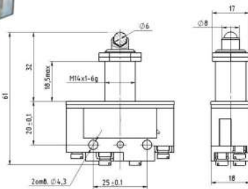
МП45-21-20511-00УХЛ3
