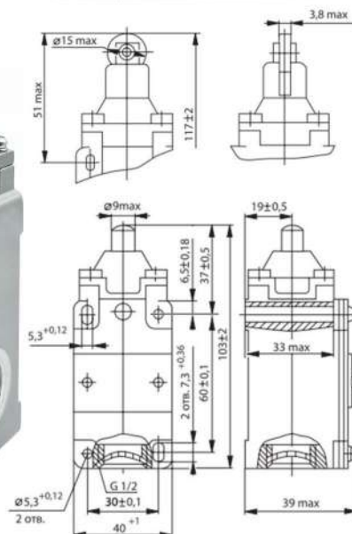
ВП15К21А221-54У2.3(У2.8) толкатель с роликом
