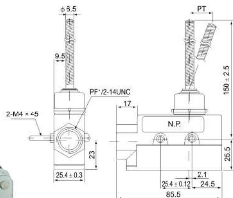
МП 45-21-10911-54УХЛ3, пружинный рычаг
