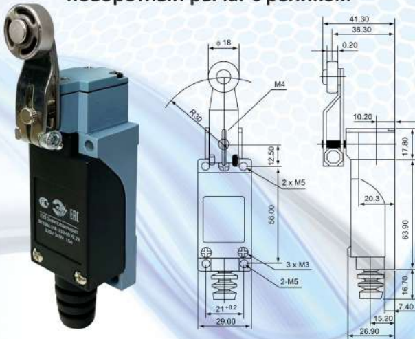
ВП19М21Б233-65 У2.28 поворотный рычаг с роликом
