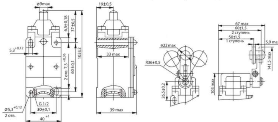
ВП15К21А231-54У2.3(У2.8) поворотный рычаг с роликом
