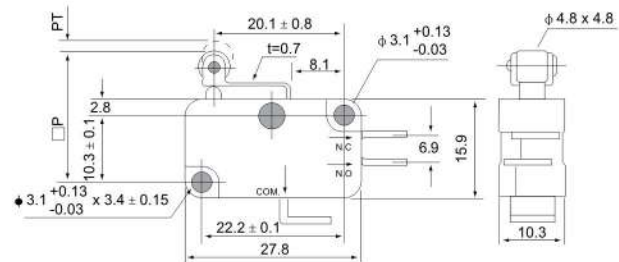
МП45-22-10913-00УХЛ3 рычаг
