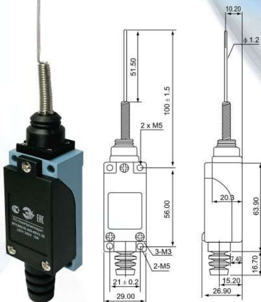
ВП19М21Б263-65 У2.28 пружинный рычаг (кошачий ус)
