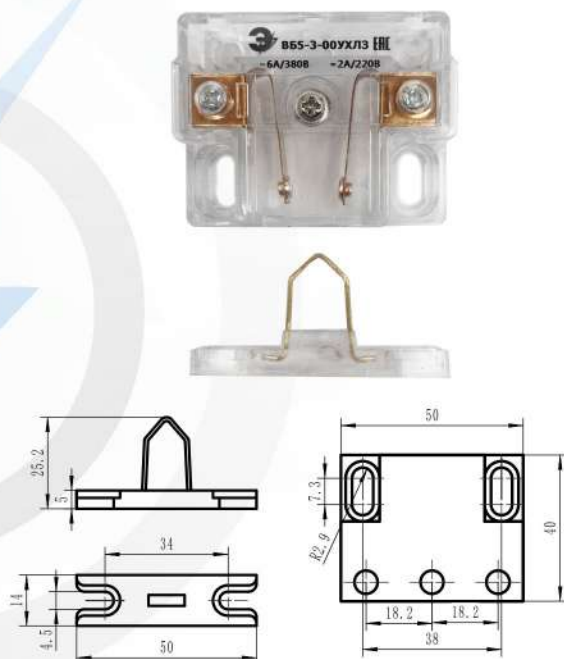
ВБ5-3-00УХЛ3
