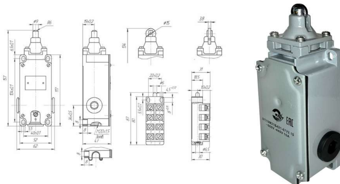
ВП19М21Б421-67У2.1Х, толкатель с роликом
