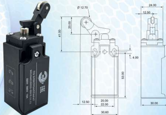
ВП19М21Б392-65У2.11(12,14) Ф поворотный регулируемый рычаг с роликом
