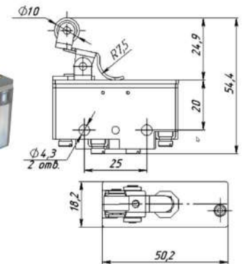
МП45-21-20911-00УХЛ3
