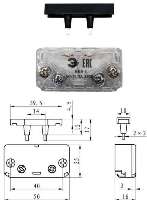
ВБ5-4-00УХЛ3
