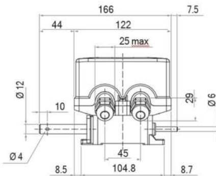
ВП19М20Б4(6)В3-65У2.2Ас(Х) с соосным валом
