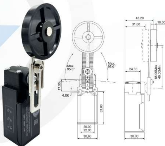
ВП19М21Б392-65У2.11(12,14)33 поворотный регулируемый рычаг с резиновым колесом
