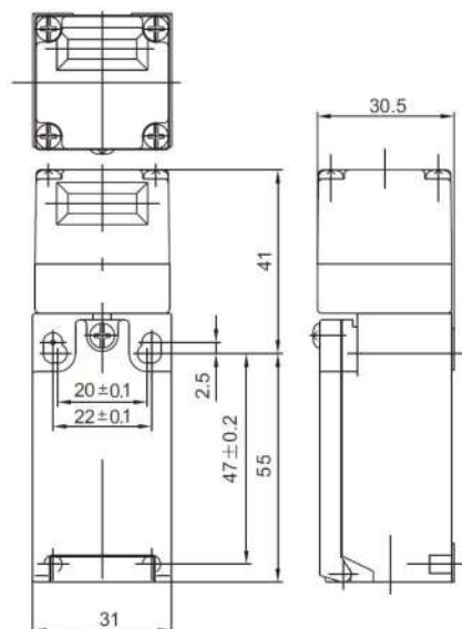
ВП19М21Б372-65У2.11(12,13,14)
