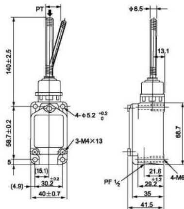
ВП15К21А241-66У2.3 пружинный рычаг с диэлектриком
