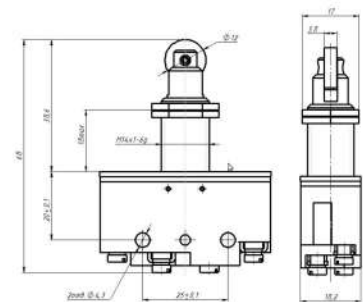
МП45-21-20611-00УХЛ3
