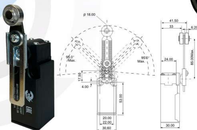
П19М21Б292-65У2.18(10,19,28) поворотный регулируемый рычаг с роликом
