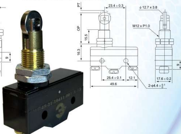
МП 45-21-10711-00УХЛЗ, короткий рычаг с роликом
