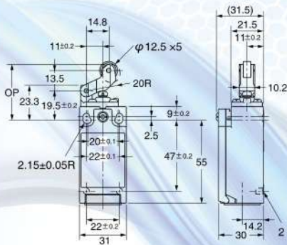
ВП31М21Б251-66У2.11(12,21,22) поворотный рычаг с роликом
