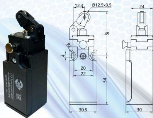
ВП19М21Б242-65У2.18(10,19,28) пружинный рычаг с диэлектриком
