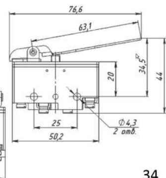
МП45-21-20911-00УХЛ3
