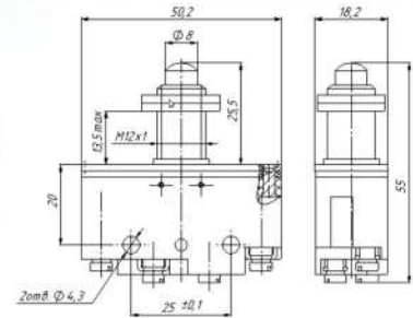
МП45-21-20411-00УХЛ3
