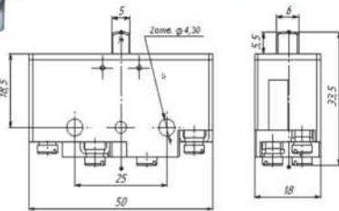
МП45-21-20311-00УХЛ3
