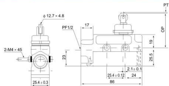
МП 45-21-10411-66УХЛ3, толкатель с роликом
