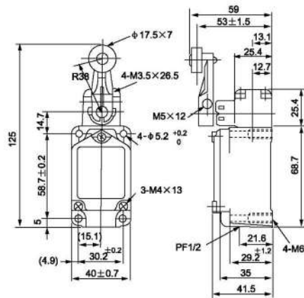
ВП15К21А231-66У2.3 поворотный рычаг с роликом
