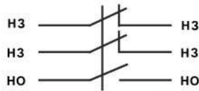
1НО+2НЗ (11)
