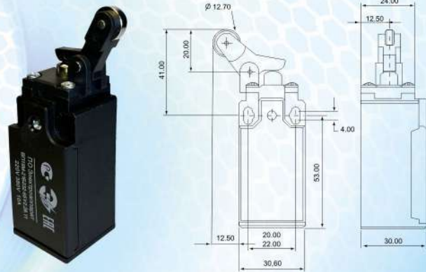
ВП19М21Б232-65У2.18(10,19,28).21 поворотный рычаг с роликом
