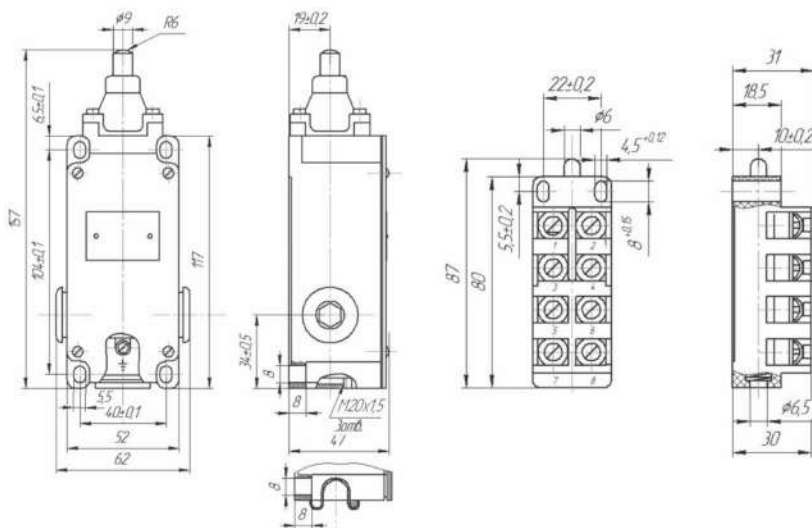
ВП19М21Б411-67У2.1Х, толкатель
