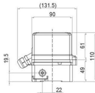
ВП19М20Б4(6)В3-65У2.2Ас(Х) с соосным валом
