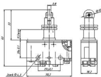
МП45-21-20711-00УХЛ3
