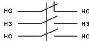
2НО+1НЗ (12)
